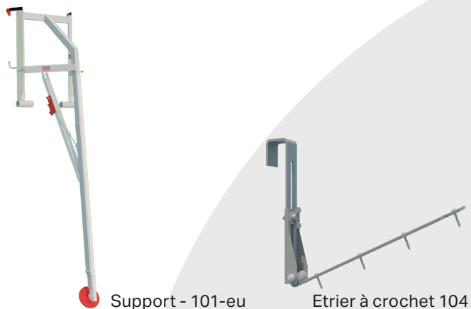
Etrier à crochet 104
